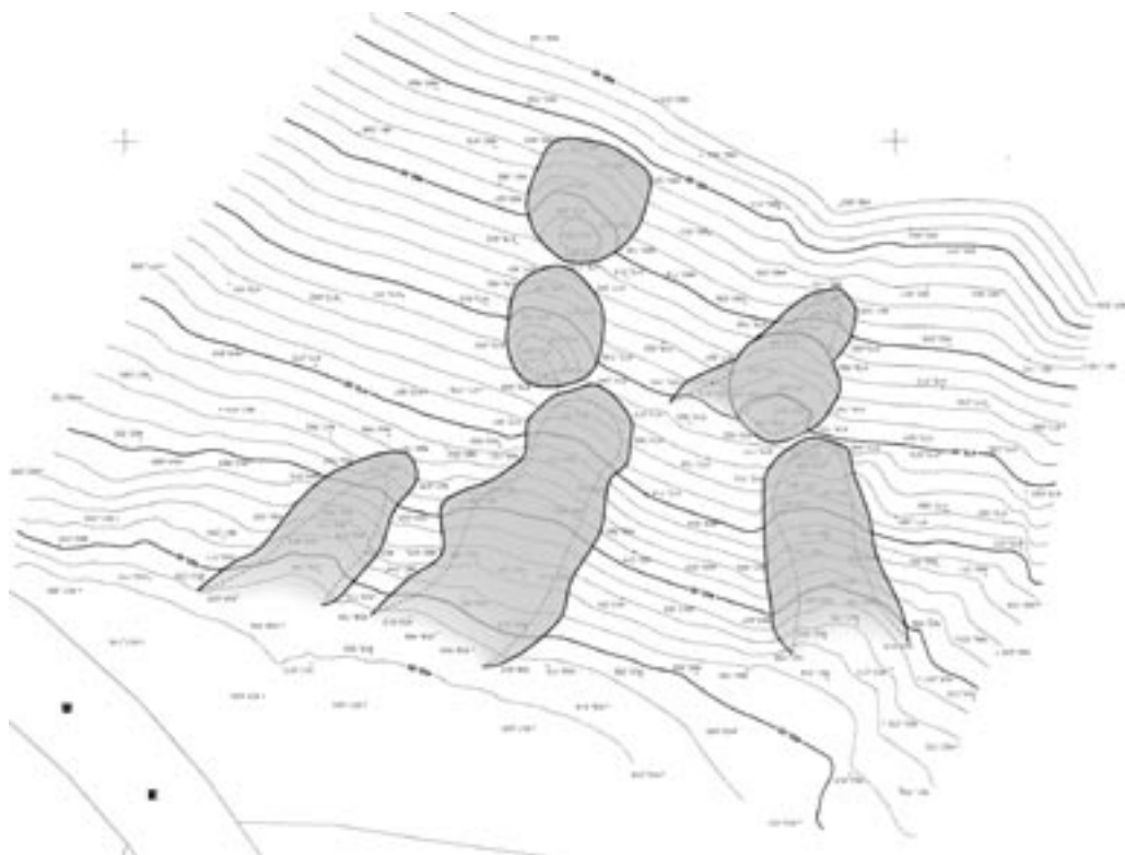
横穴塚陥没跡測量図
