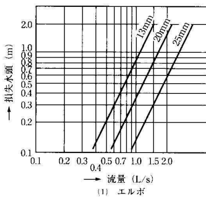
図II-5-12 管継手部の損失水頭図
