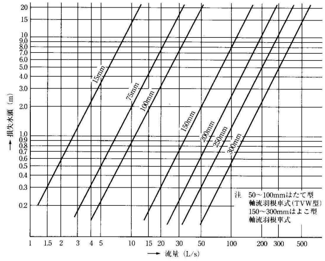
図II-5-11 大口径メータの損失水頭図
