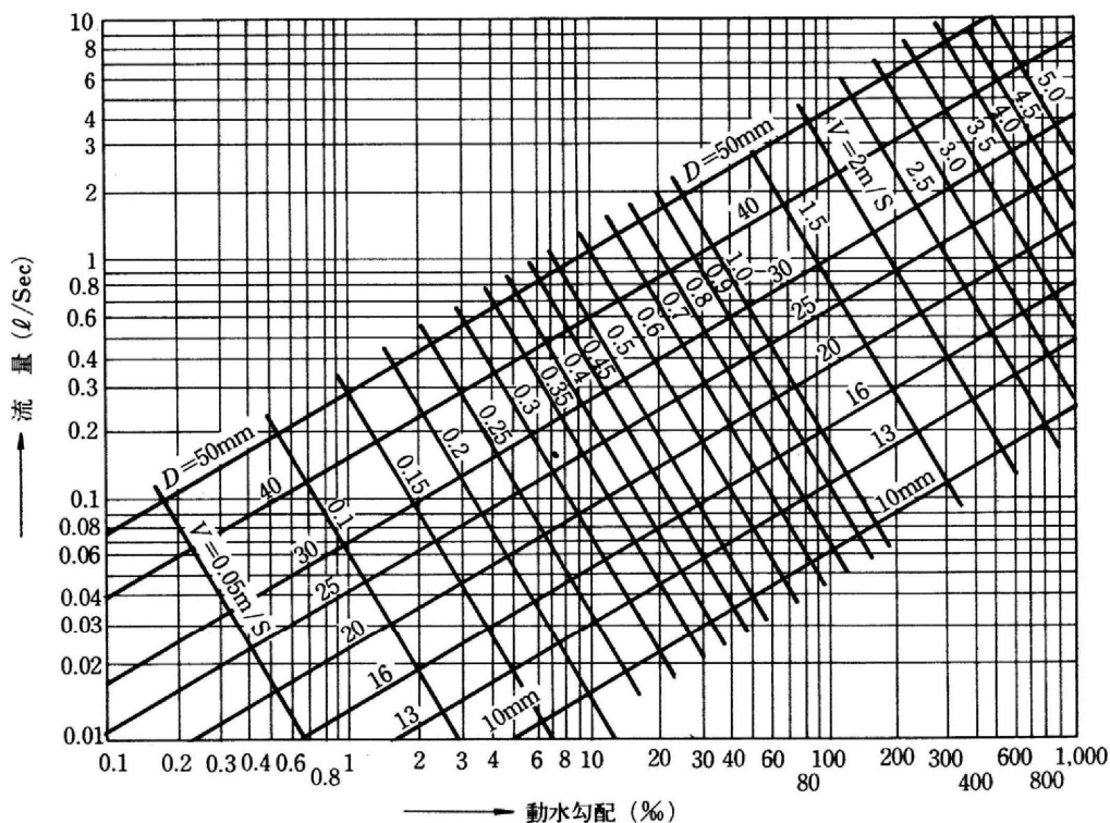
図Ⅱ-5-4 ウェストン公式による給水管の流量図
