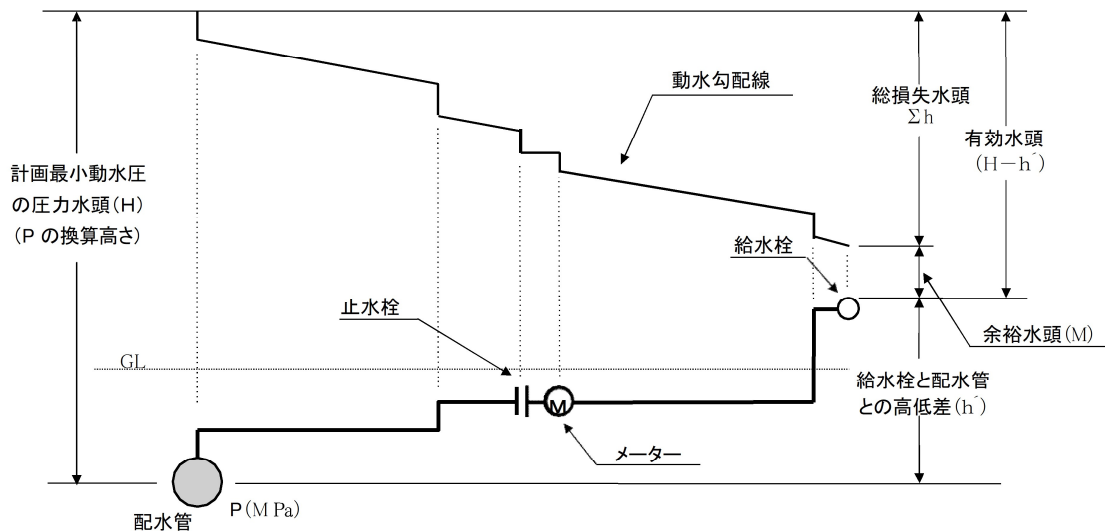
図Ⅱ-5-2 動水勾配配線図
