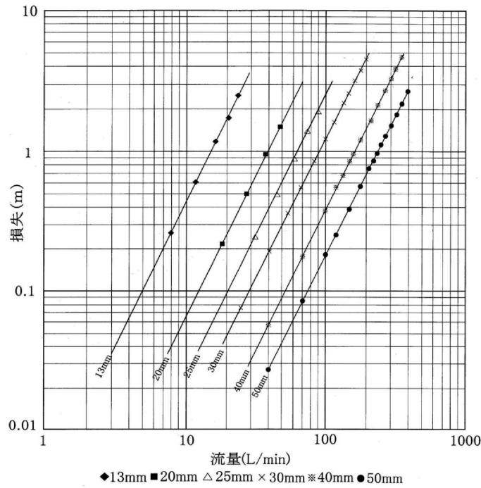
図Ⅱ-5-7 サドル分水栓の損失水頭図
