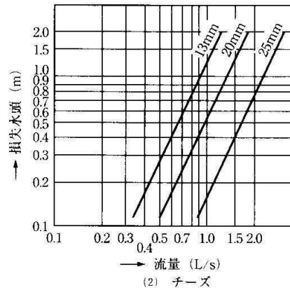
図II-5-12 管継手部の損失水頭図
