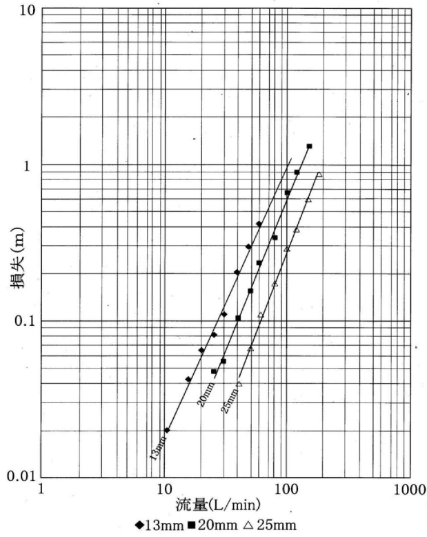
図 II-5-9 ボール止水栓の損失水頭図
