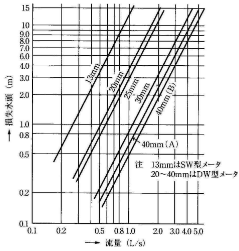
図II-5-10 メータの損失水頭図
