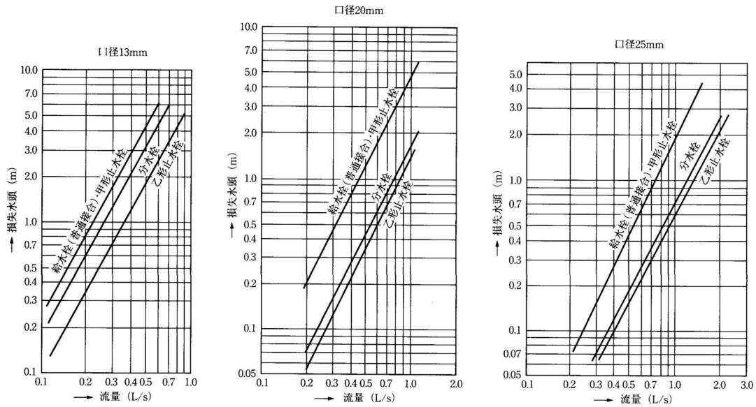
図Ⅱ-5-6 給水栓、止水栓、分水栓の損失水頭
