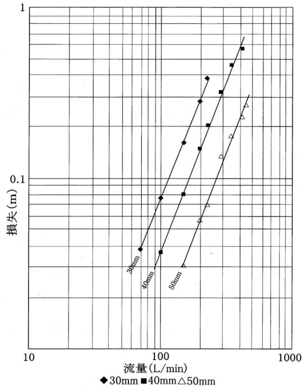
図 II-5-8 青銅製ソフトシール弁の損失水頭図
