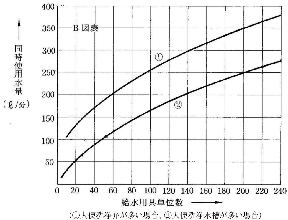
図 II-5-1 同時使用水量
