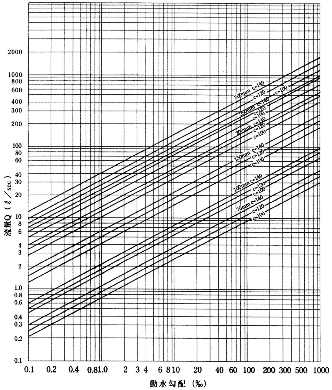
図Ⅱ-5-5 ヘーゼン・ウィリアムス公式流量図
