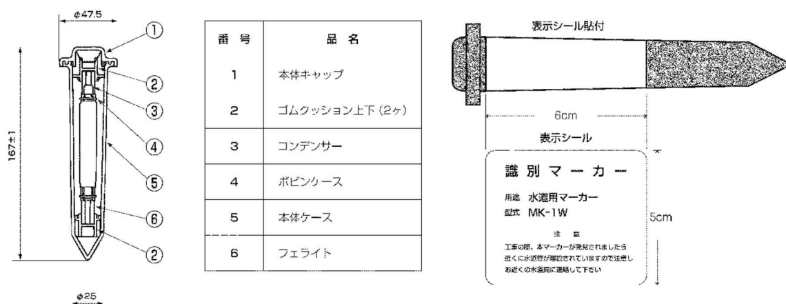
写真Ⅲ-7-3 水道用識別マーカ－
