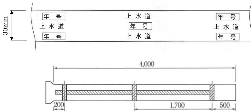
図Ⅲ-7-1 明示テープ設置例
