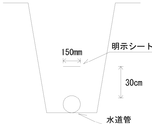
図Ⅲ-7-2 明示シート文字例及び標準施工図
