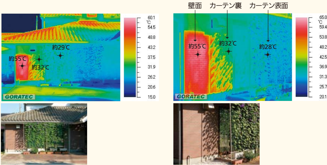
カーテン裏と壁面の温度差23℃
