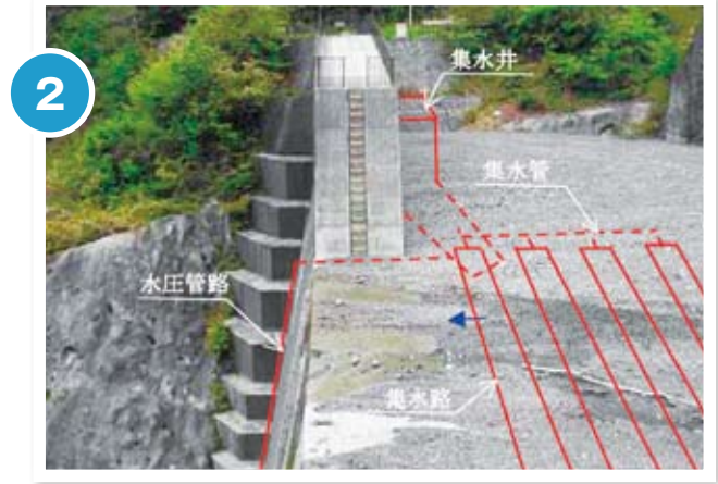
金山沢川砂防えん堤 集水地周辺
