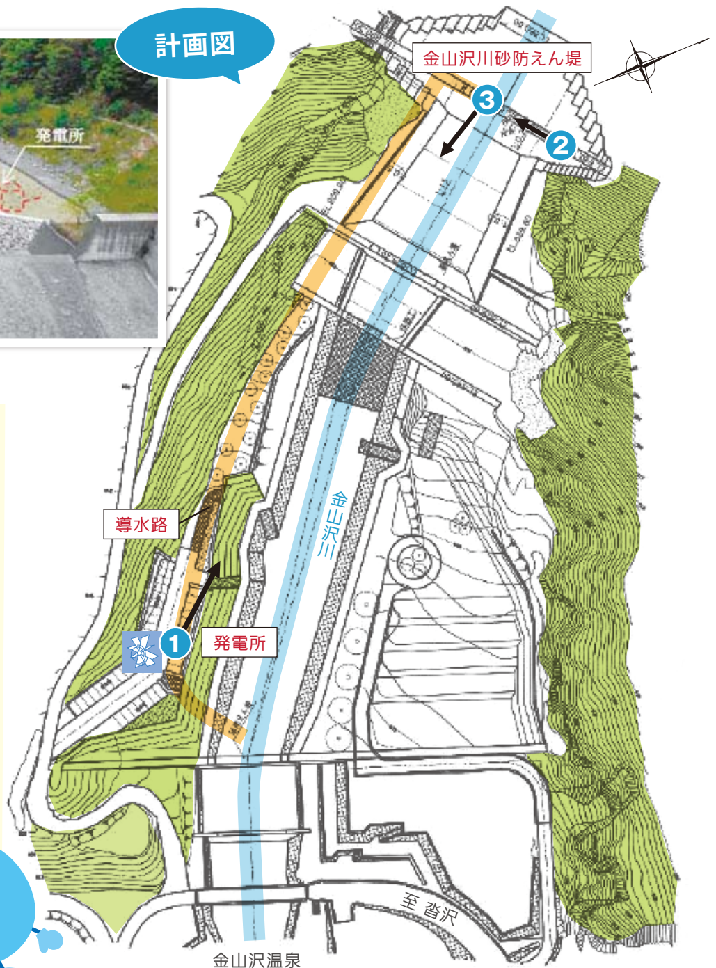
金山沢川砂防えん堤 集水地周辺
