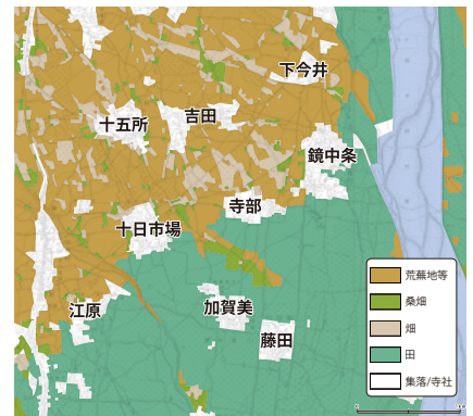
明治21年の土地利用状況：御勅使川扇状地扇端部の鏡中条、寺部、十日市場、江原あたりの湧水線を境に、その北側が荒地か畑地、その南が水田となっていることがわかる。
