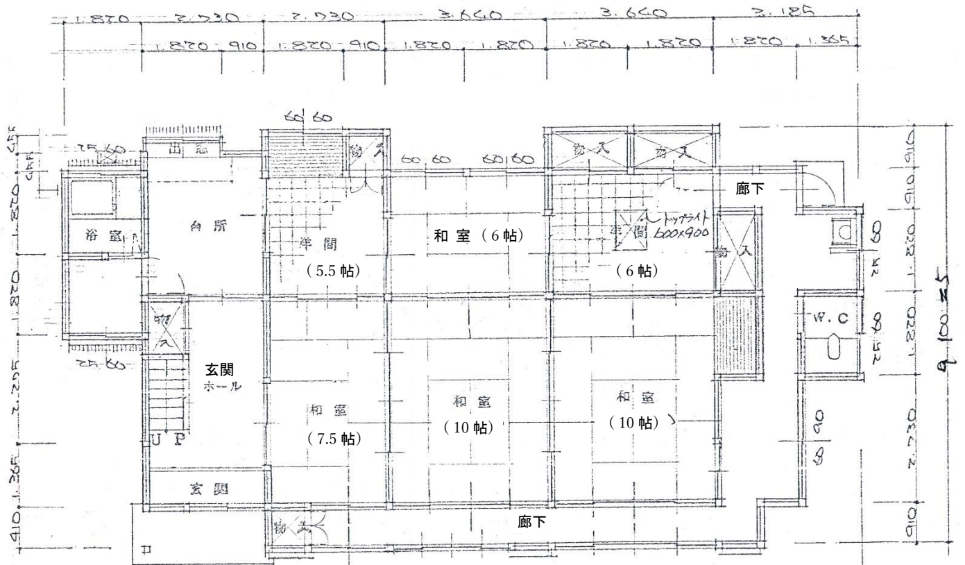
1階 平面図
